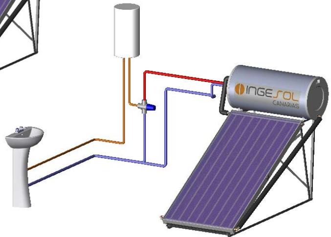
Termosifón con válvula mezcladora y termo de apoyo
