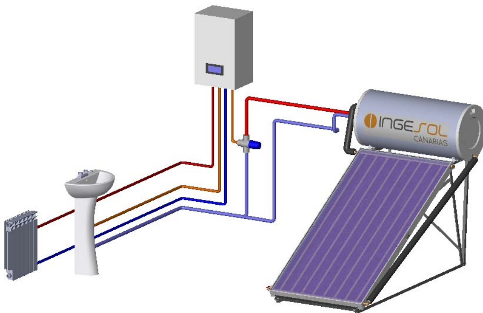
Termosifón válvula mezcladora y caldera
