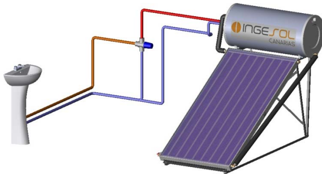
Termosifón con válvula mezcladora
